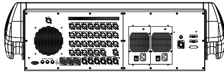
リアパネル
