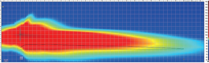
VLSシリーズの音響シミュレーション例 (VLS30: 垂直指向角度 +3° ~ -11°)
