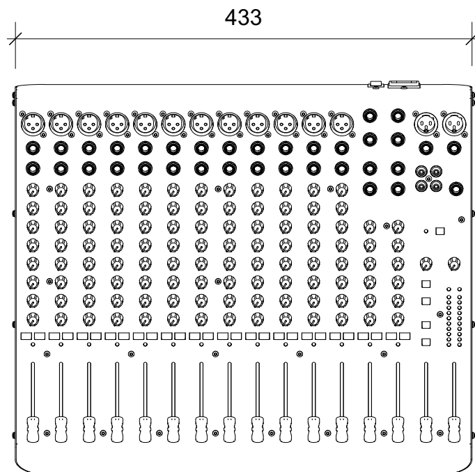
TOP
