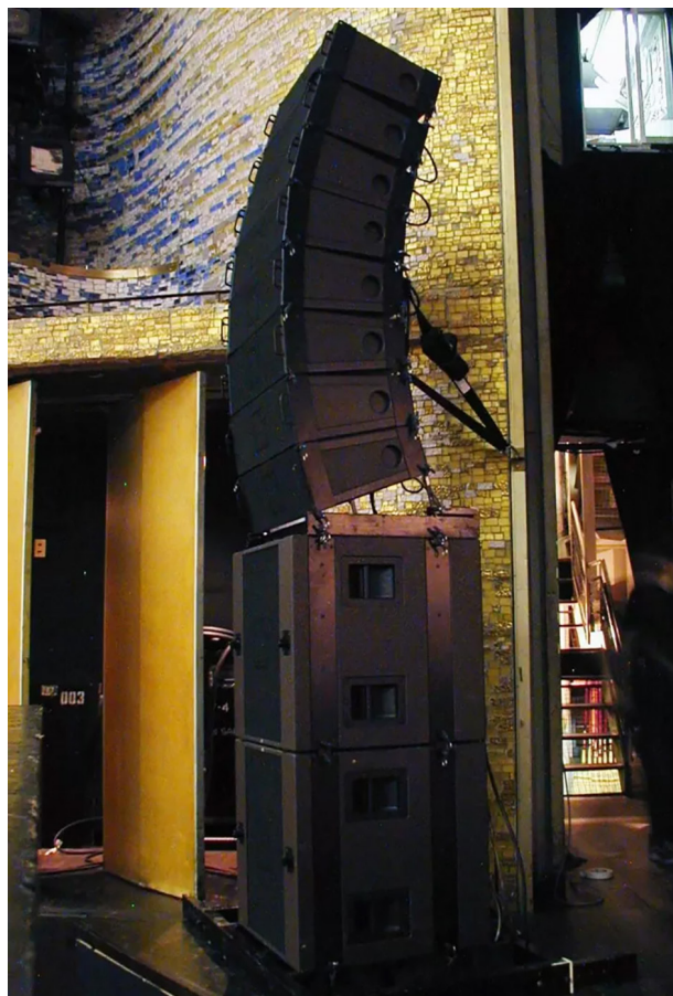
dV-DOSCとdV-SUBのグランドスタック
