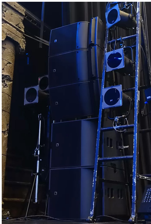
サイドスピーカーとして使用したA15 Focus とKS21
