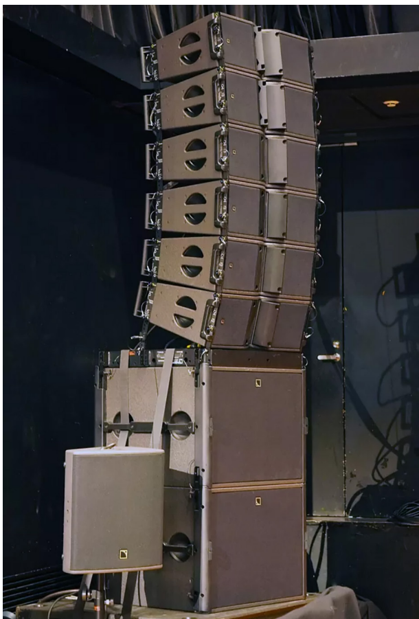
Kara(KaraII にアップグレード済) とSB18のグランドスタック
