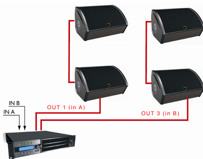
図 4 : 115XT HiQ 4 台を LA4 コントローラー 1 台に接続する
