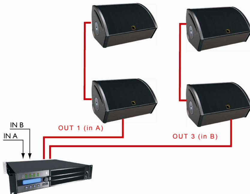
図 5：115XT HiQ 4 台を LA4 コントローラー 1 台に接続する
